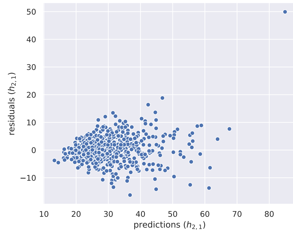
Residual Plot (w/ proj. spaces)
