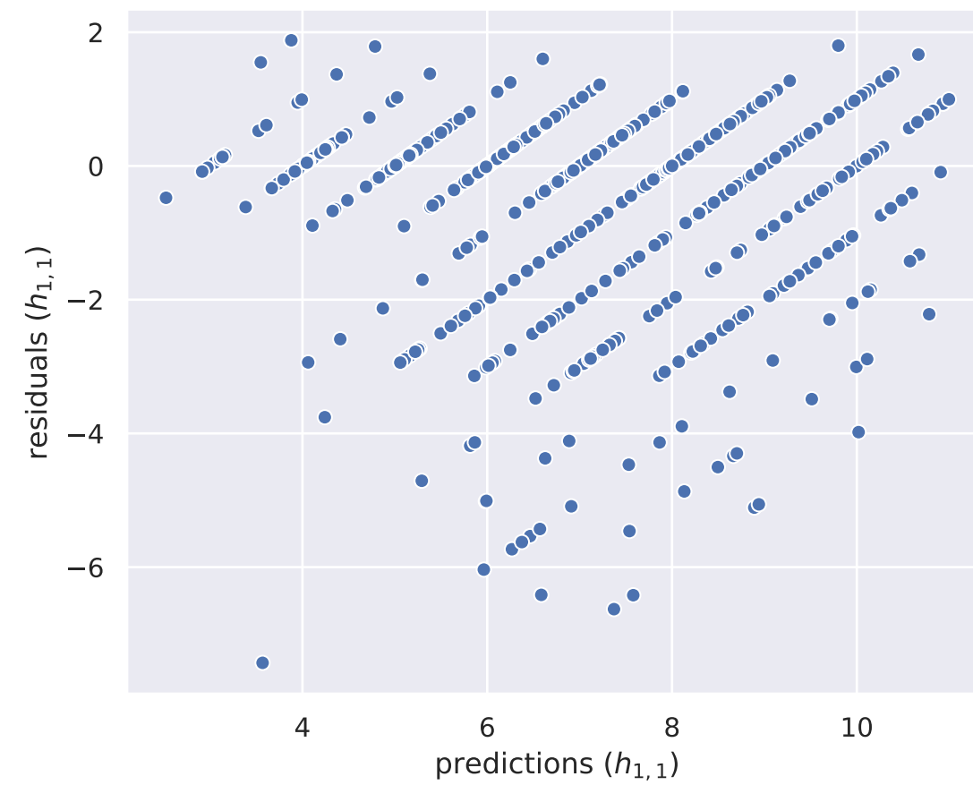
Residual Plot (w/ proj. spaces)
